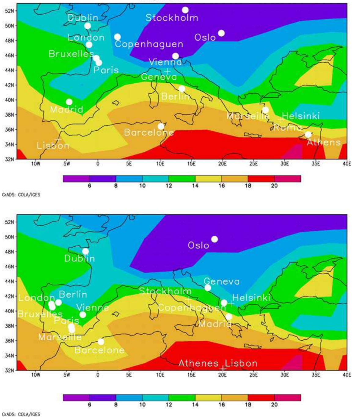
Figur 12 Angivelse af det bedste analoge klima til en række byer baseret på to klimamodeller. En cirkel indikerer at analogen er baseret på både temperatur og nedbør, mens et kryds indikerer, at det ikke har været muligt at finde en sådan analog. Krydset markerer da den bedste analog baseret på temperaturen (Hallegatte et al, 2007).
